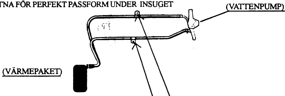
PLÅTKLAMMREN SOM HÅLLER VÄRMEPAKET SLANGARNA. SÅ DOM EJ TAR MOT INSUGETS FÖRVÄRMNINGSKANAL. DESSA VIKTIGA PLÅTBITAR SAKNAS VÄLDIGT OFTA. SKRUVAS FAST MED INUGSBULTARNA. 1955-62 MED SLANGARNA UNDER INSUGET.
